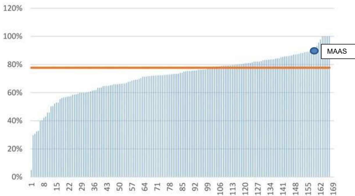
Figura 3.12. Rendiment de la xarxa per als serveis analitzats. El valor mig és 78%. Gràfic núm. 6 Rendiments de les xarxes analitzades a l'estudi de l'ASAC
